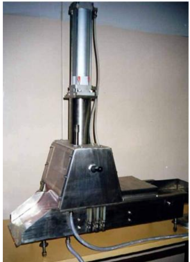
Рис. 6 Пневматичний ін'єктор-автомат Я5-ФШ1Л (розробка фахівців ППР НААН)
